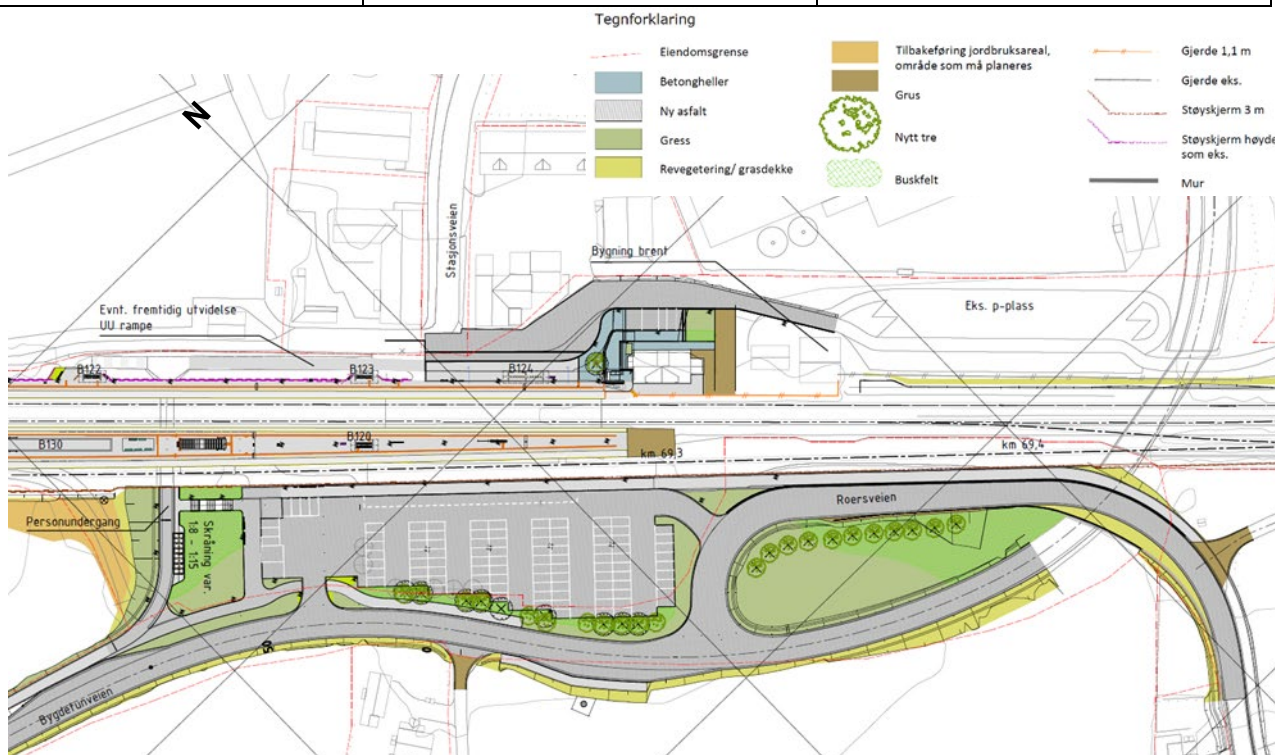
Figur 12 Oversiktsskisse som viser utforming av parkeringsplass og sidearealer på sørvestsida av sporene på Rygge stasjon (Tegning ICH-11-O-25107). I plankartet er det i tillegg innarbeidet plass til forlengelse av busslommene og leskur ved busslommene i Bygdetunveien.
