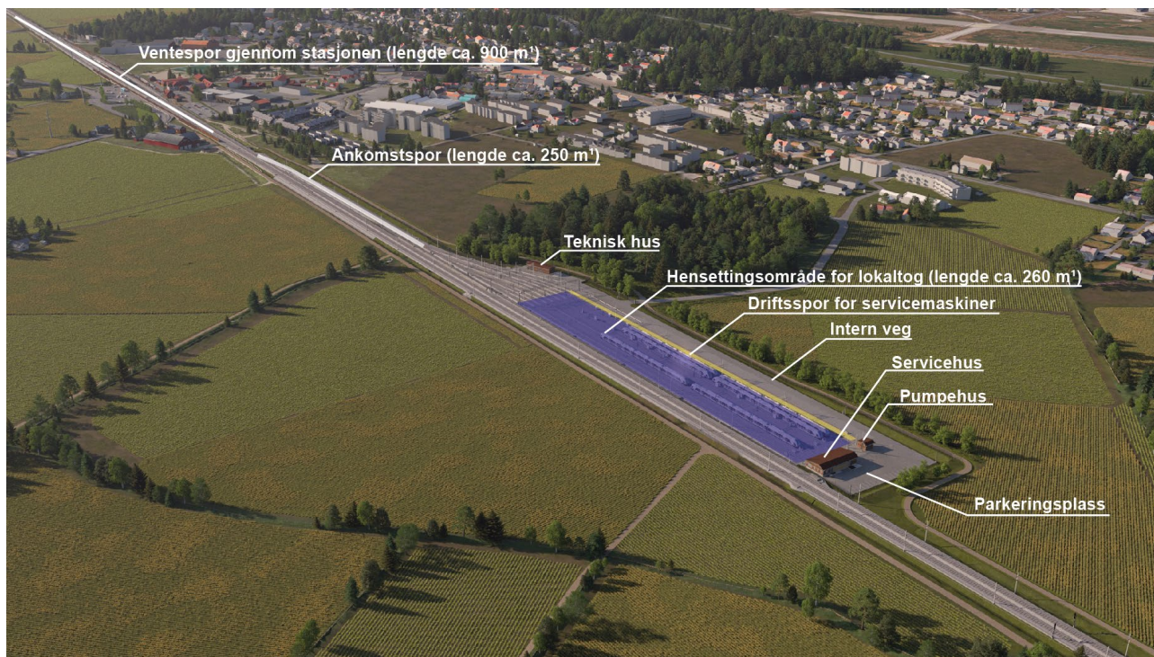
Figur 2 Prinsippskisse av hensettingsanlegget, med plassering av noen viktige elementer. 1) lengder er oppgitt som tilgjengelig sporlengde for tog.
