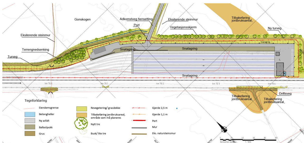
Figur 15 Oversikt over hensettingsanlegget med Trafikkarealer, sideareal og vegetasjonsetablering. (Tegning ICH-11-O-25102).
